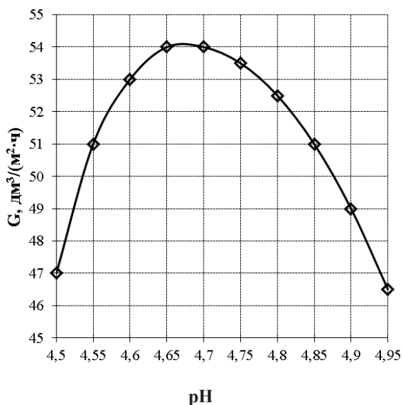
Рис. 12. Зависимость проницаемости УФ мембран от активной кислотности творожного калье при u = 3,0 м/с; P = 0,35 МПа, t = 55 °C; C = 12\% СВ, мембрана КУФЭ (0,01)
