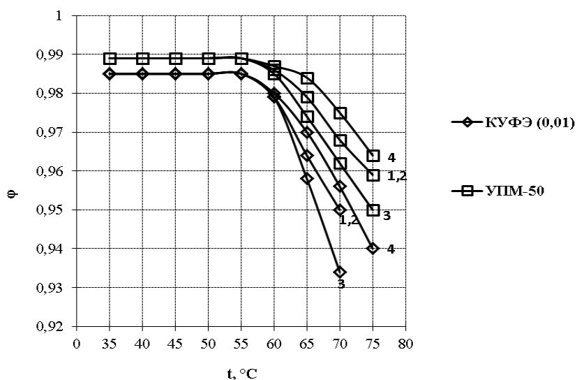
Рис. 11. Зависимость селективности УФ мембран от температуры (творожное калье) при u = 3,0 м/с; P = 0,35 МПа. 1 - C = 17\% СВ; 2 - C = 15\% СВ; 3 - C = 20\% СВ; 4 - C = 12\% СВ
