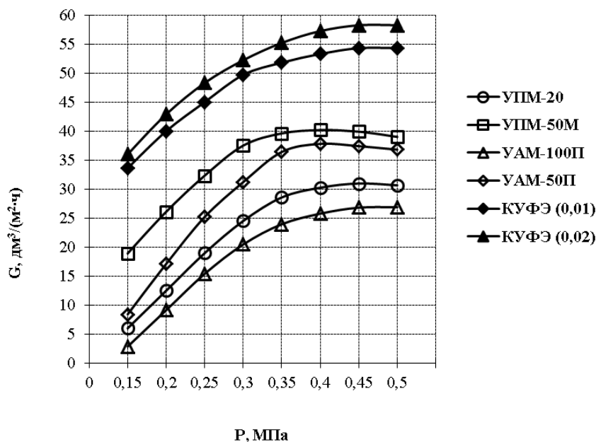
Рис. 5. Зависимость проницаемости УФ мембран от давления (творожное калье) при u = 3,0 \text{ м/с} ; t = 55 \text{ }^\circ\text{C} ; C = 12 \text{ \% СВ}
