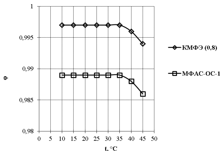
Рис. 10. Зависимость селективности МФ мембран от температуры (обезжиренное молоко) при u = 4,5 м/с; P = 0,25 МПа; C = 8,5 % СВ
