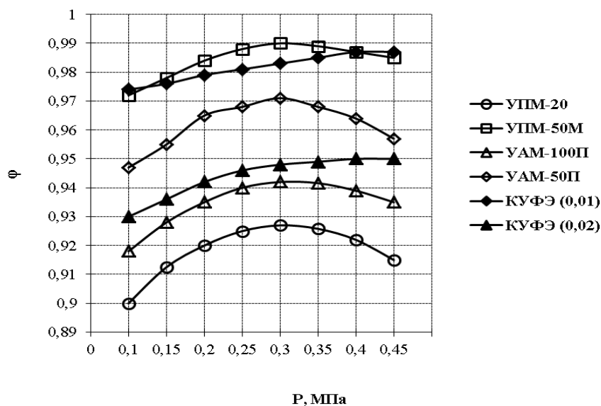
Рис. 7. Зависимость селективности УФ мембран по белкам от давления (творожное калье) при u = 3,0 \text{ м/с} ; t = 55^\circ\text{C} ; C = 12\% \text{ СВ}
