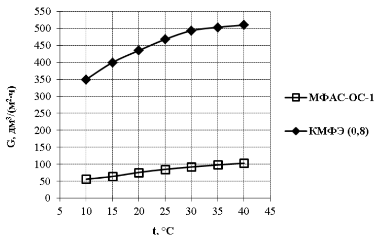
Рис. 8. Зависимость проницаемости МФ мембран от температуры (обезжиренное молоко) при u = 4,5 м/с; P = 0,25 МПа; C = 8,5 % СВ
