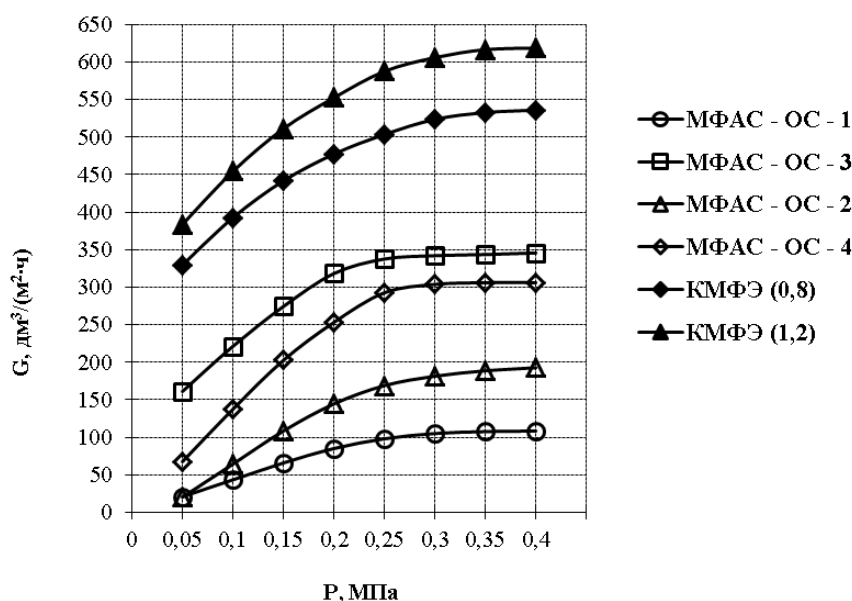
Рис. 4. Зависимость проницаемости МФ мембран при разделении обезжиренного молока от давления при u = 4,5 м/с; t = 35 °C; C = 8,5 % СВ
