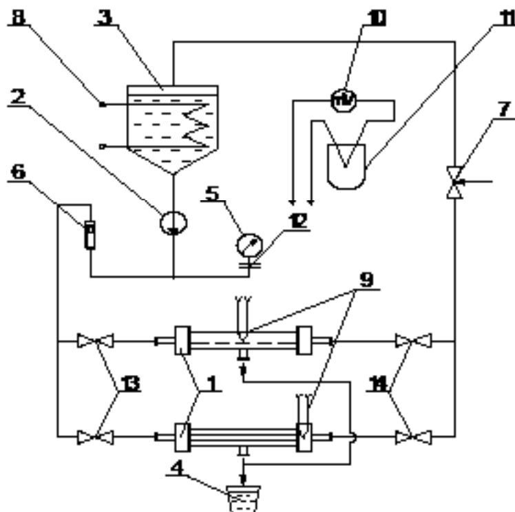
Рис. 1. Схема лабораторной установки для исследования процессов МФ и УФ.
