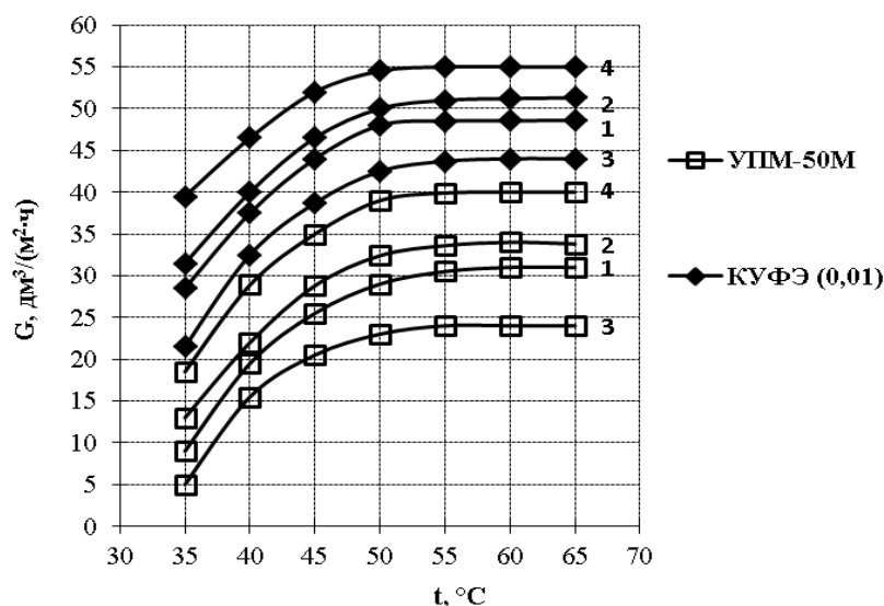
Рис. 9. Зависимость проницаемости УФ мембран от температуры (творожное калье) при u = 3,0 м/с; P = 0,35 МПа. 1 – C = 17\% СВ; 2 – C = 15\% СВ; 3 – C = 20\% СВ; 4 – C = 12\% СВ
