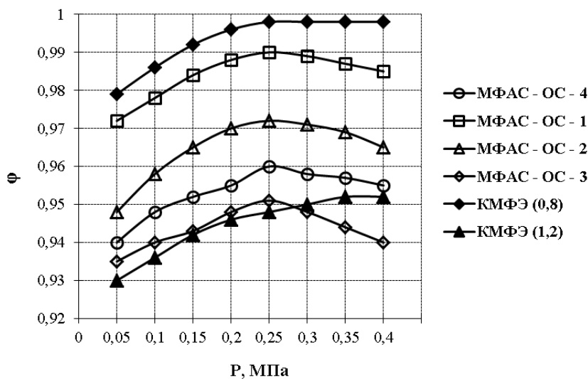
Рис. 6. Зависимость селективности по микрофлоре МФ мембран при разделении обезжиренного молока от давления при u = 4,5 \text{ м/с} ; t = 35 \text{ }^\circ\text{C} ; C = 8,5 \text{ \% СВ}
