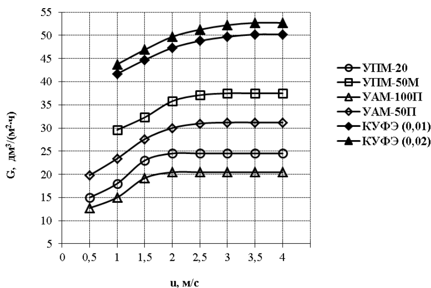
Рис. 3. Зависимость проницаемости УФ мембран от скорости течения творожного казеина над мембраной при P = 0,3 МПа; t = 55 °C; C = 12 % СВ
