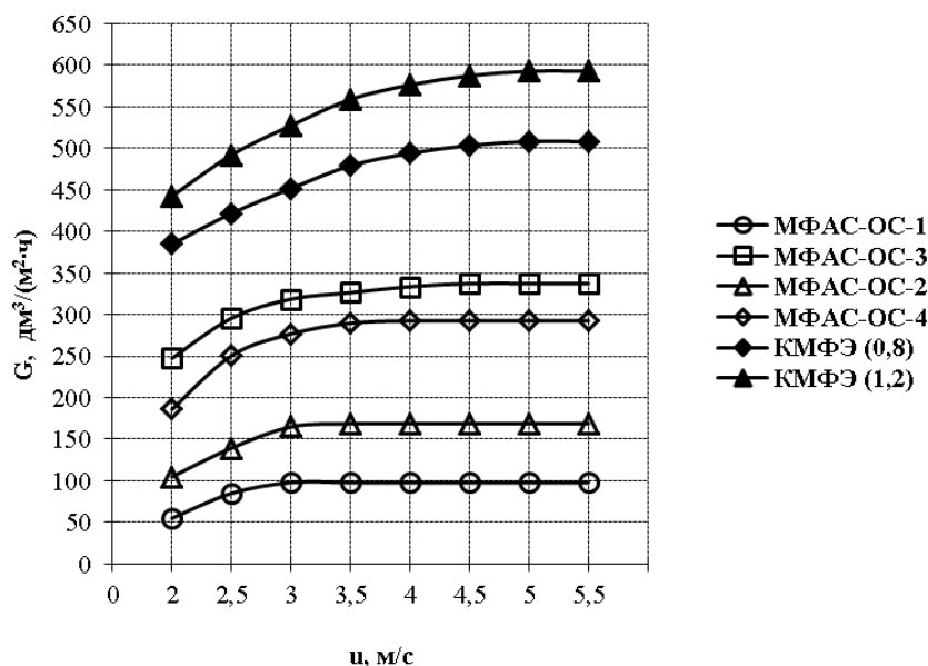
Рис. 2. Зависимость проницаемости МФ мембран от скорости течения обезжиренного молока над мембраной при P = 0,25 МПа; t = 35 °C; C = 8,5 % СВ
