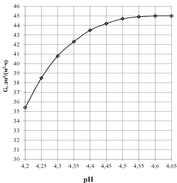
Рис. 13. Зависимость проницаемости УФ мембраны от активной кислотности УФ творога при u = 3,0 м/с; P = 0,35 МПа, t = 55 °С; C = 15,0 % СВ, мембрана КУФЭ (0,01)
