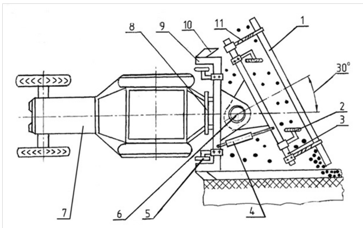
Рис. 1. Принципиальная схема агрегата для сбора и утилизации камней в горной местности: 1 – гребенка, 2 – опорные колеса гребенки, 3 – подвижная рама, 4 – гидроцилиндр, 5 – опорные колеса плуга, 6 – поворотное устройство, 7 – трактор МТЗ-82, 8 – навесное устройство, 9 – неподвижная рама, 10 – корпус плуга, 11 – пружинные стойки
