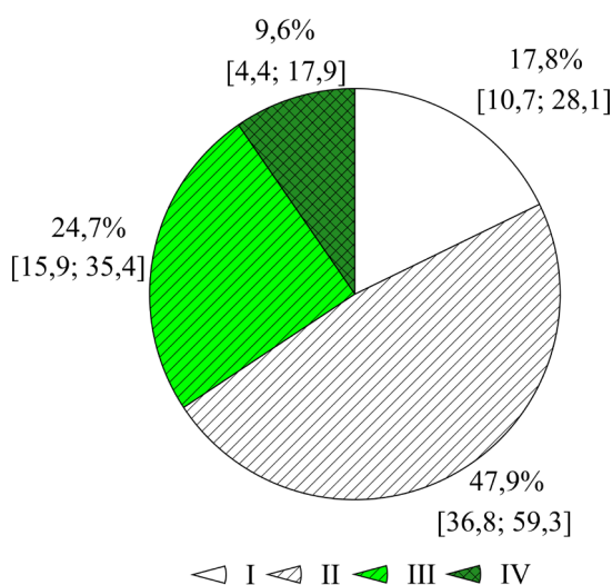
Рис. 5. Распределение подземных вод Сосновского района Челябинской области по категориям качества
