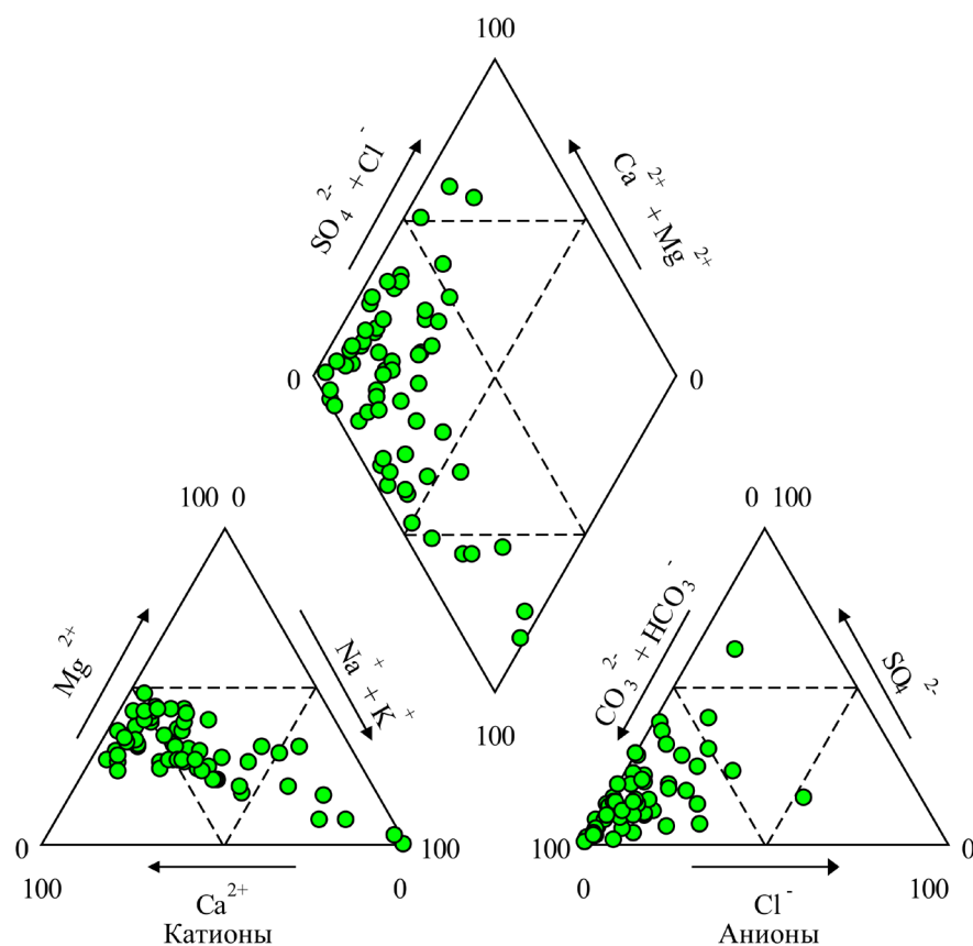
Рис. 2. Подземные воды Сосновского района на диаграмме Пайпера
