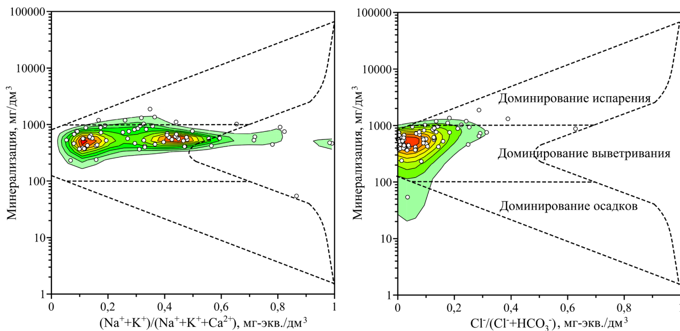
Рис. 4. Подземные воды Сосновского района Челябинской области на диаграмме Гиббса
